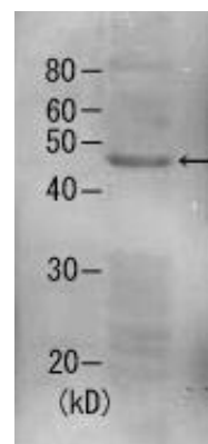
図 1 S. cerevisiae 粗抽出液においてこの抗体を用いてウェスタンブロットィングを行い、Rpn7 (49kDa)を検出した。
